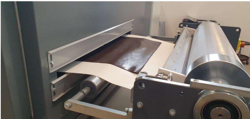
Fase di asciugatura di uno dei campioncini testati dopo applicazione del fondo bio
